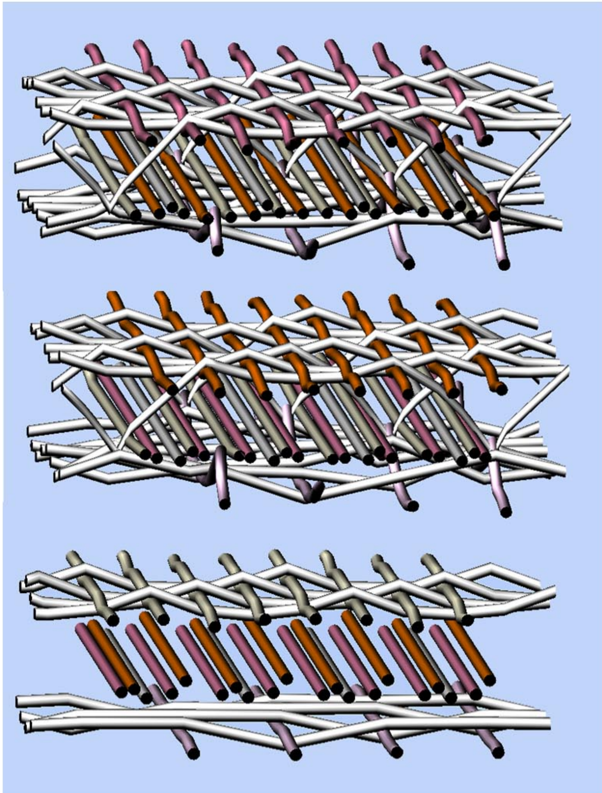
HÁROM SZÍN//RÉTEG ÁBRA//KÖTÉSRAJZ
