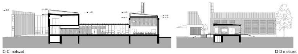
C-C metszet
