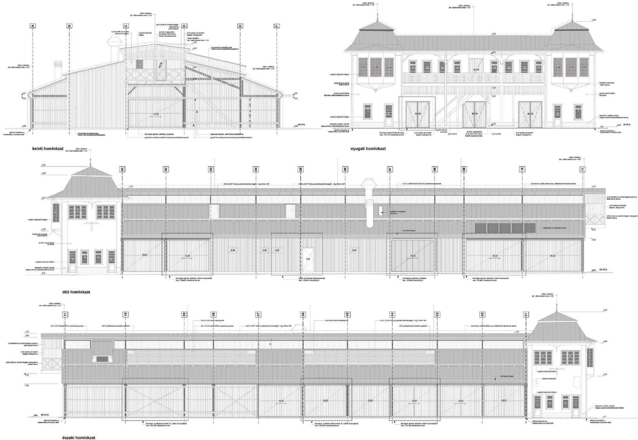
A III. Csónakház homlokzatai
