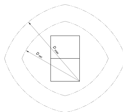
A legnagyobb látótávolság szerkesztése 60
