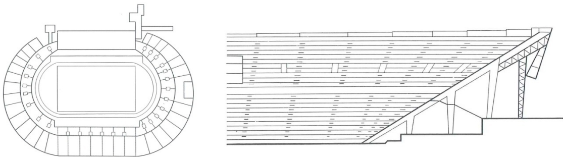
Olympiastadion Helsinki, Yrjo Lindegren, Toivo Jantti, 1938, alaprajz és jellemző metszet az ideiglenes tribünnel 50
