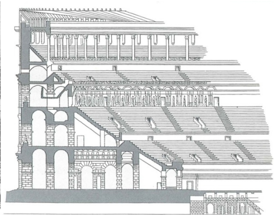
A római Amphiteatrum Flavium metszete 17
