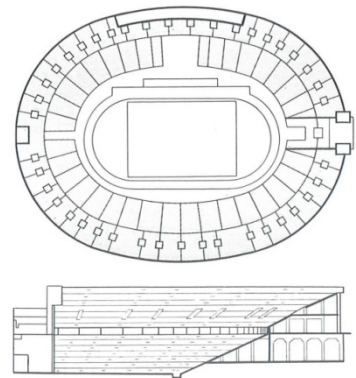
Alaprajz és jellemző metszet 47
