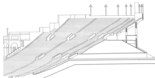
A Coliseum földdombra épített nagyvonalú metszete 56
