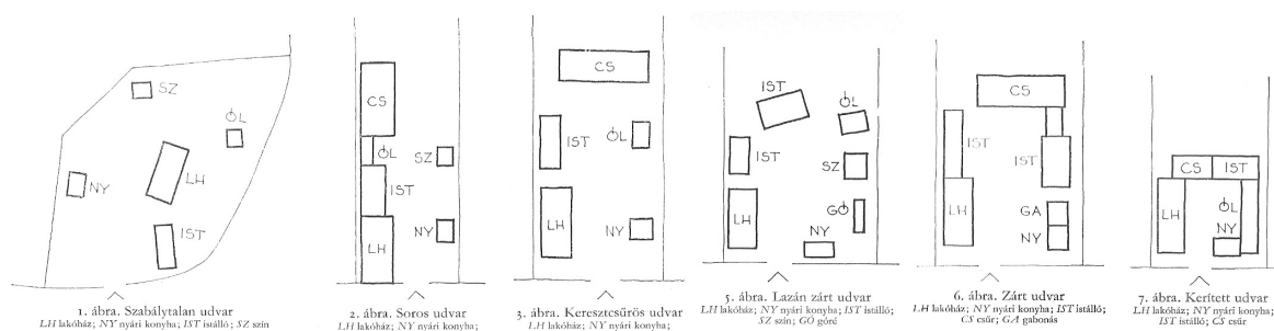
19. kép: főbb udvar típusok a népi építészetben, balról jobbra: szabálytalan, soros, keresztcsűrös, lazán zárt, zárt, kerített Az udvarok, mint a vidéki építészet és gazdaság alapját, keretét képező formációk, melyek megismerése és értelmezése Reischl számára a vidéki építészet alapját jelentette.
