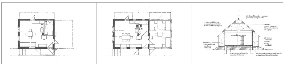
90-92. képek: “keretet adó”, fejleszthető lakóház javaslatok a beregi újjáépítésre, Reischl Gábor, 2001
